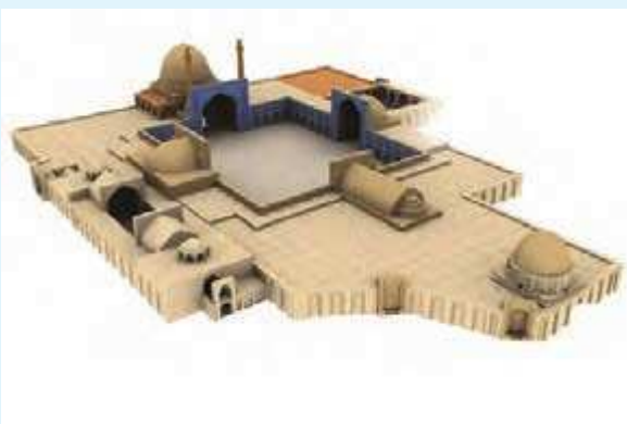
پلان کلی مسجد چهار ایوانی
