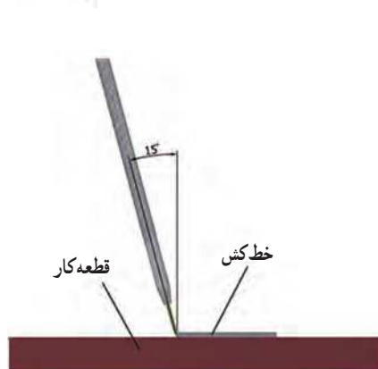
شکل ۴-۵. روش صحیح خط‌کشی با خط‌کش و سوزن خط‌کش
