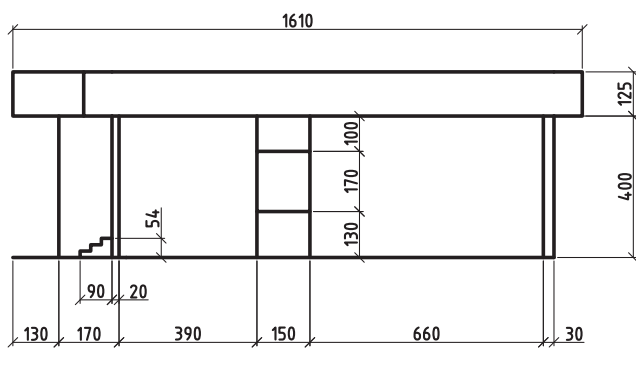
شکل ۹-۲. نقشه نماهای ساختمان
